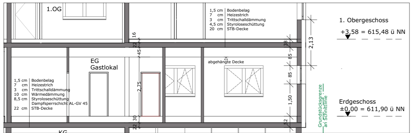
Schnitt 01
